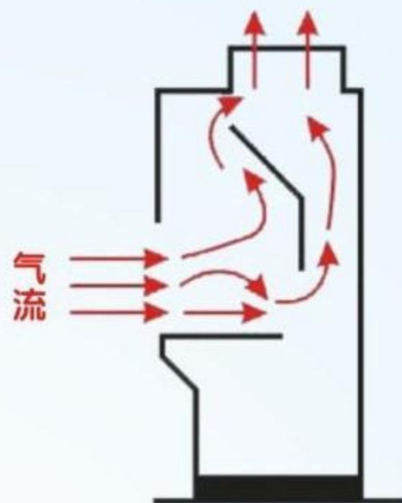
通风柜原通风原理
